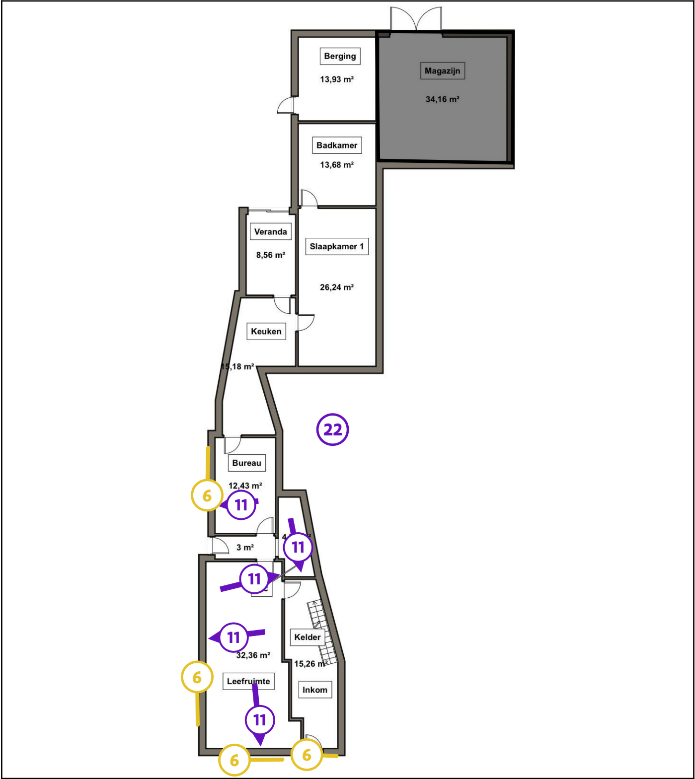
Legende van plan 1.3: Gelijkvloers 0.1
