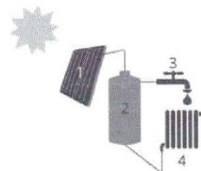
1. Zonnecollector | 2. Opslagvat zonneboiler | 3. Sanitair warm water | 4. Afgifte-element voor ruimteverwarming (optie-een)
